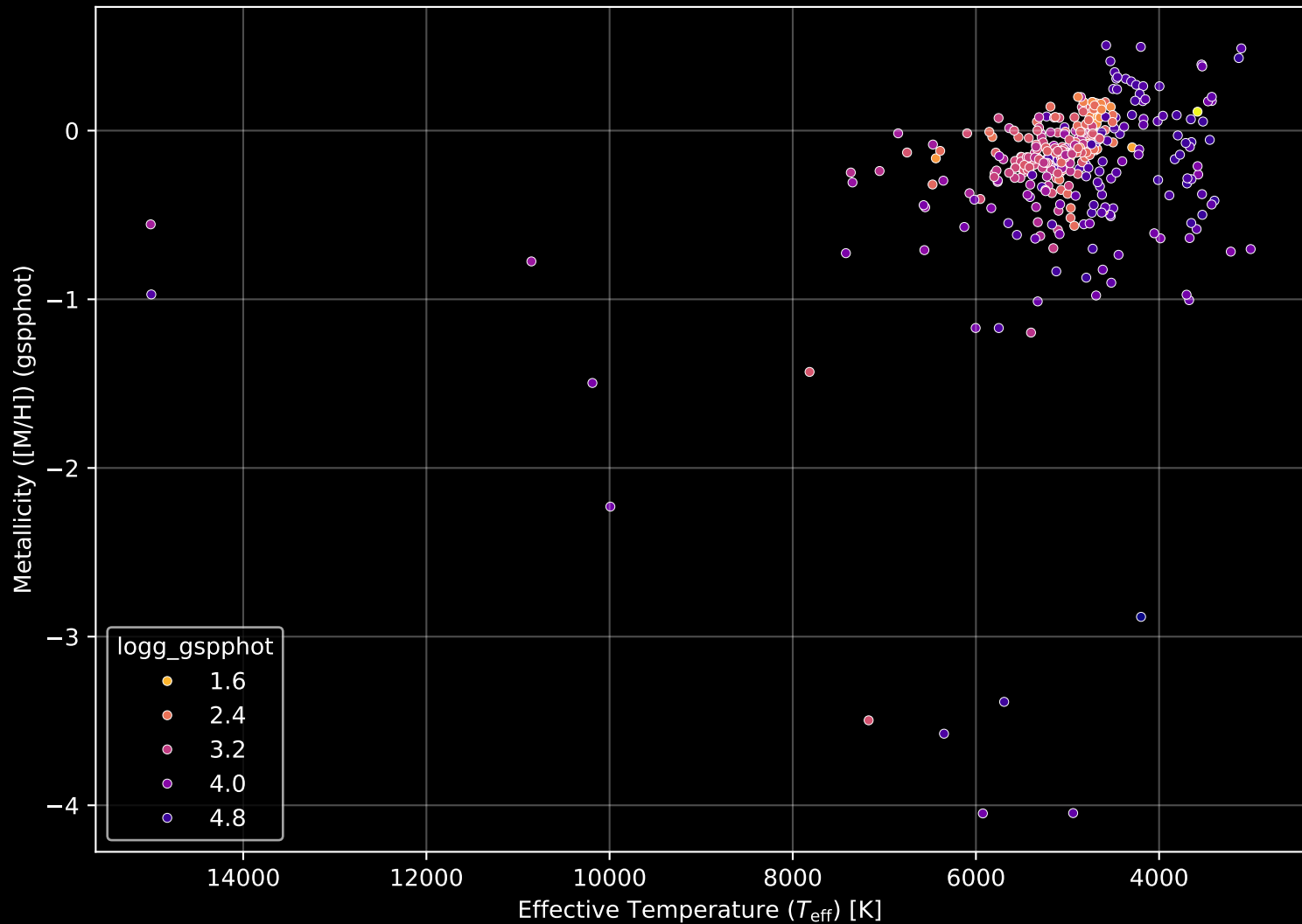
APOGEE DR17 Field: [TAUL1551_btx] Stellar Population Parameters (n= 374)
